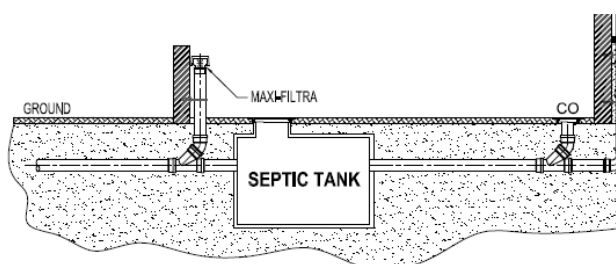
Septička jama
