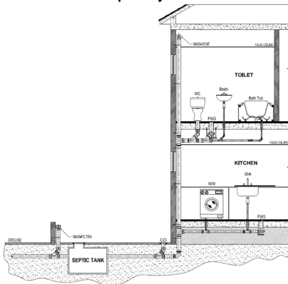
Septička jama
