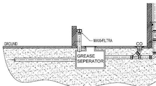
Separator
